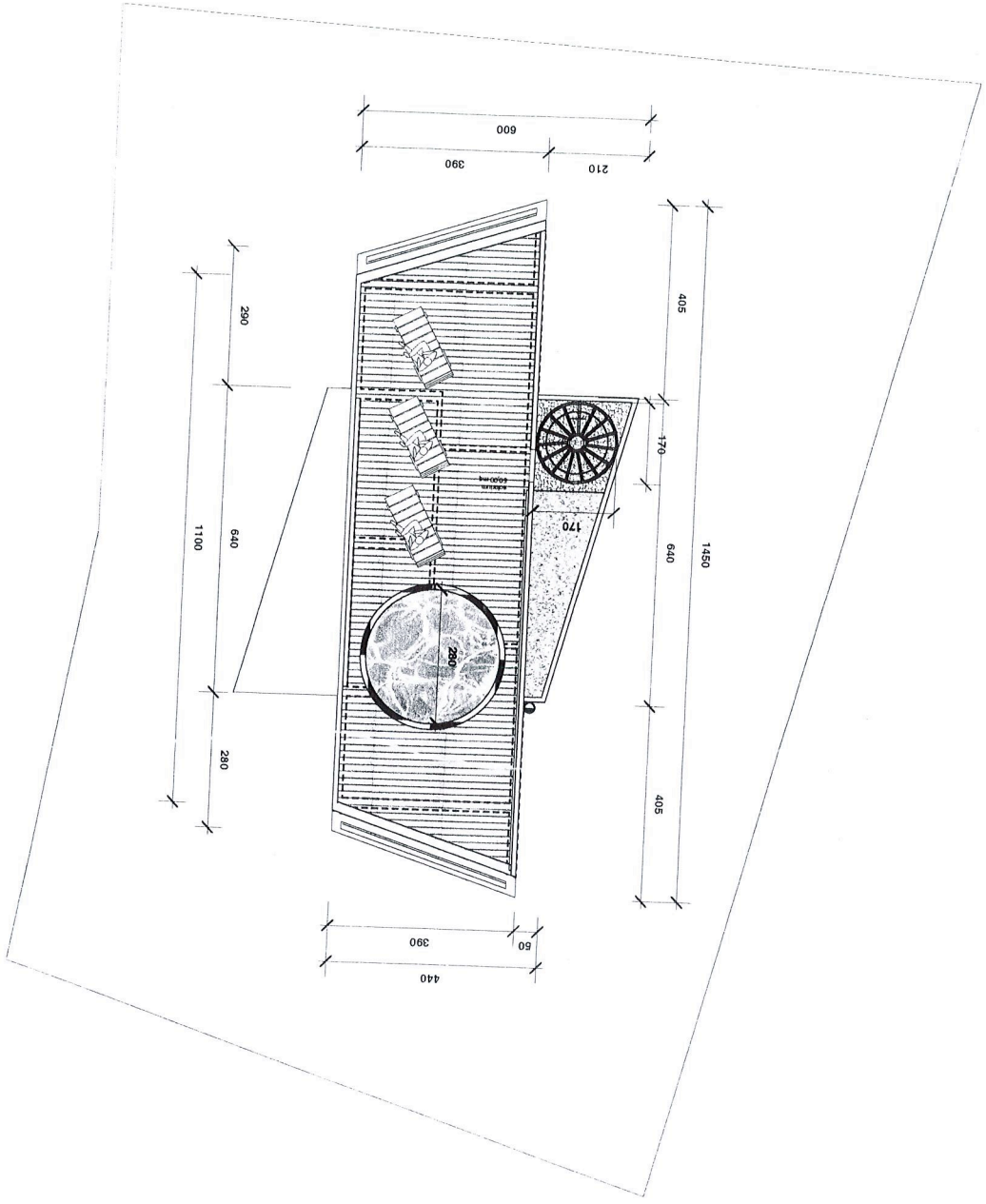
PIANTA PIANO COPERTURA
